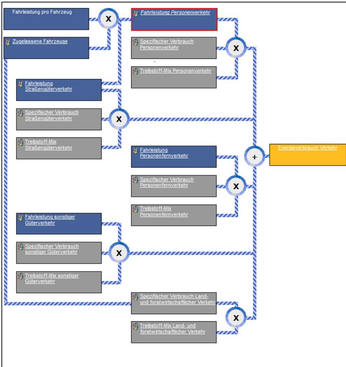
Abbildung 39: Berechnungsmodell nach ECOSPEED Region (B.A.U.M./IfE, 2015)
